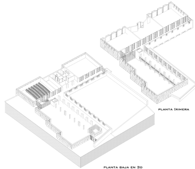
PLANTA BAJA EN 3D
