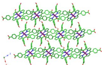
fig 2. Proyección [010] de las capas 2D unidas por enlaces de hidrógeno para [Fe(TCPP)]. (Fe-morado, O-verde, N-azul, H-grís).
