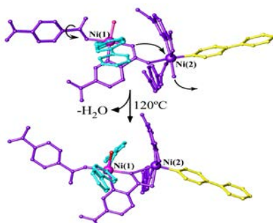
fig 1. Transformación estructural del compuesto [Ni_2(PDC)_2(bipy)_{1.5}(H_2O)_2] \cdot 3.5H_2O (1).
