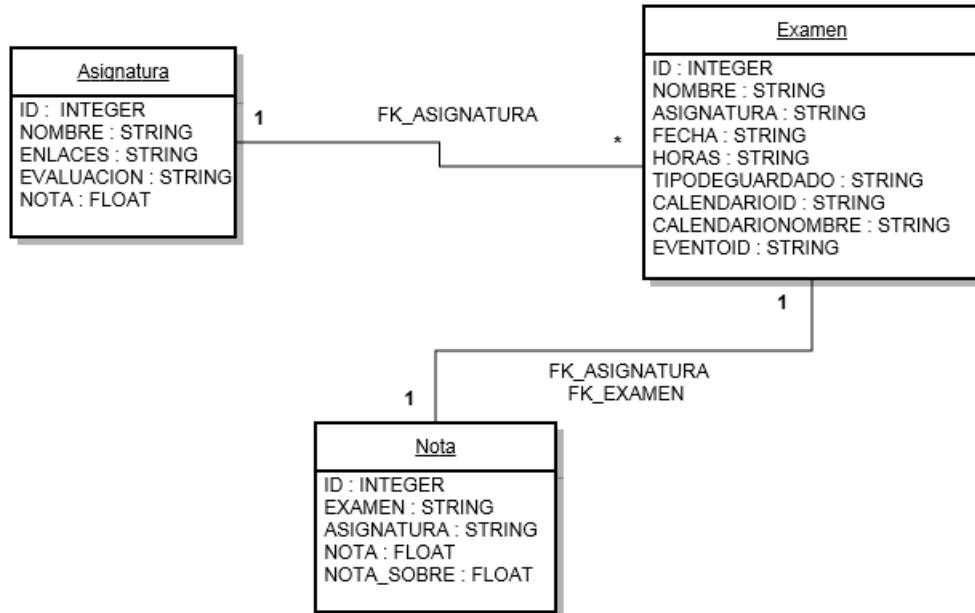
Figura 5.4: Modelo relacional
