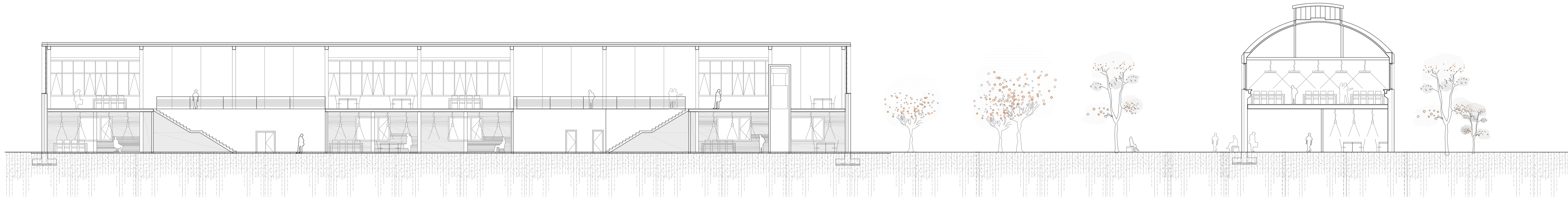
_katedral handiaren erdiko nabearen luzetarako ebaketa
