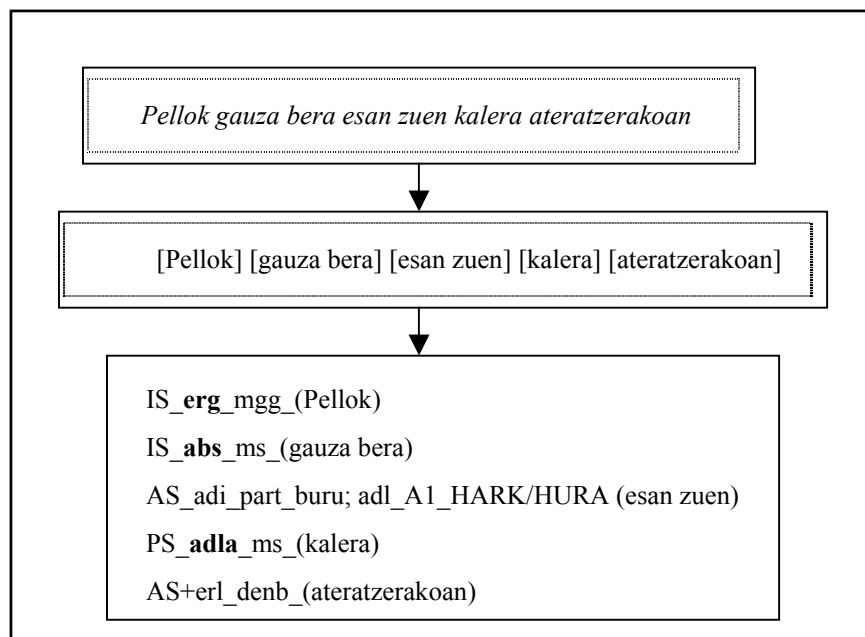
III.2 irudia. Analizatzailearen emaitzaren adibide bat.
