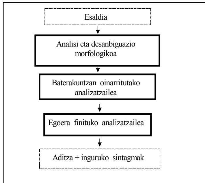
III.1 irudia: Esaldia analizatzeko sistemaren eskema orokorra.
