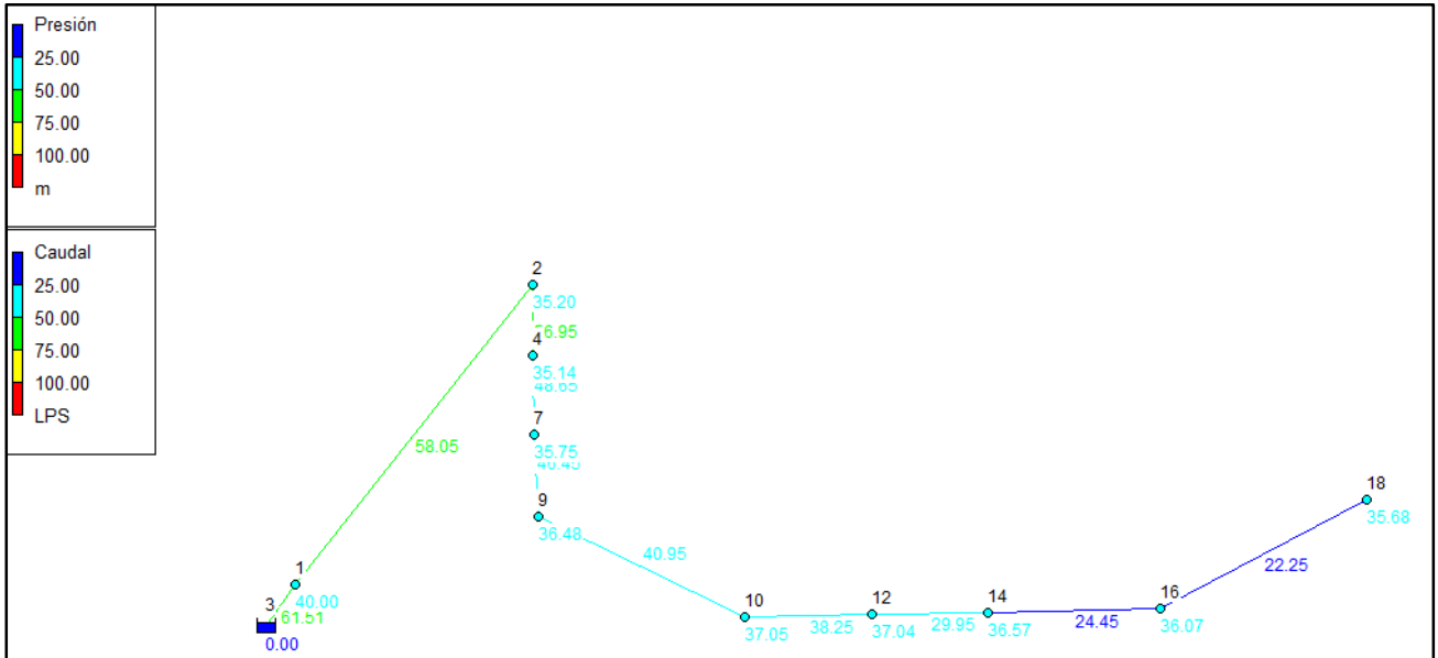
Diagrama Presión-Caudal
