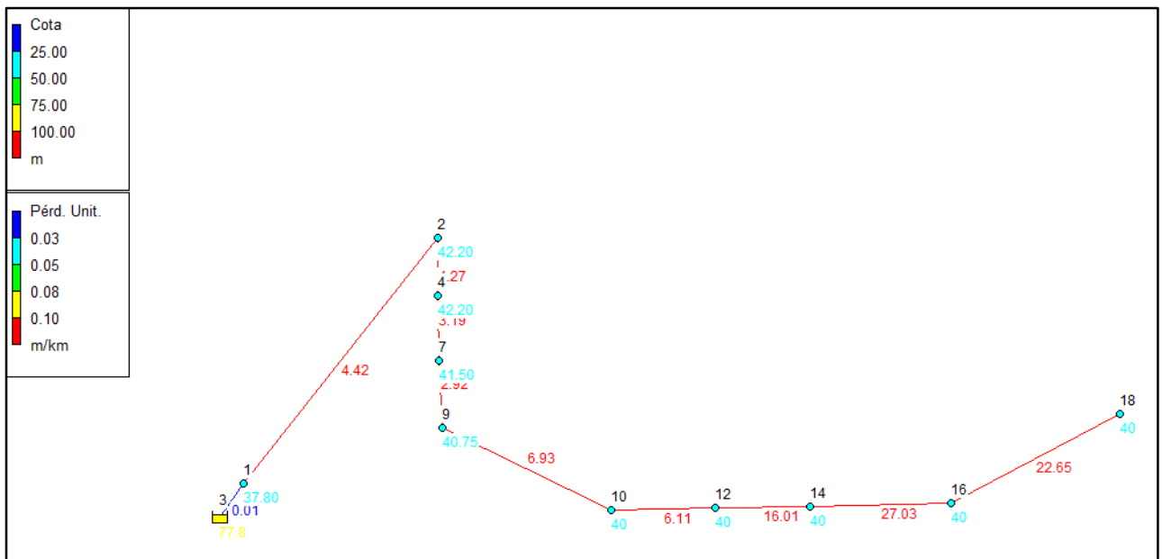
Diagrama Cota-Pérdida unitaria
