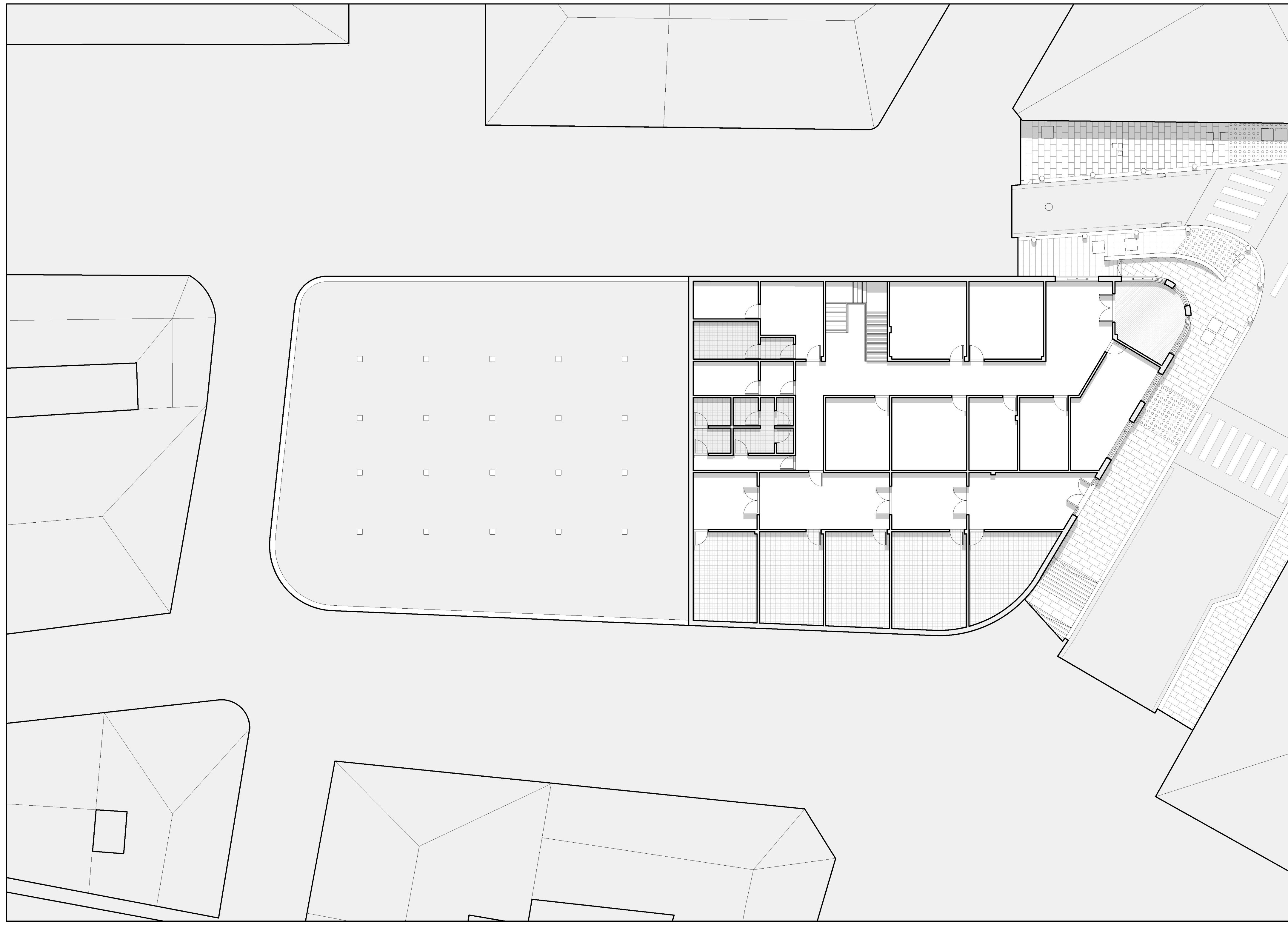
ERDISOTO SOLAIRUA Eskala 1 : 300 Portugaleteko Merkataria erdisoto solairua
