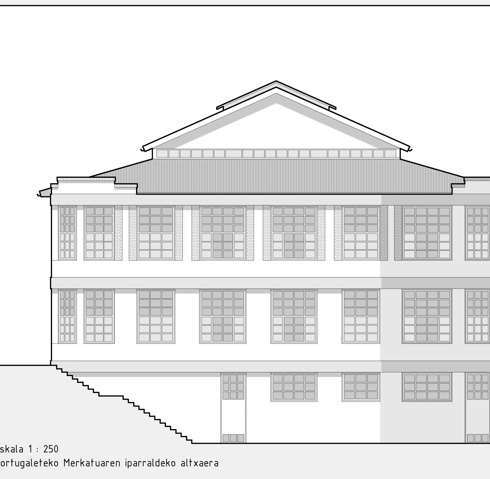
Eskala 1 : 250 Portugaleteko Merkataria iparraldeko altxaera
