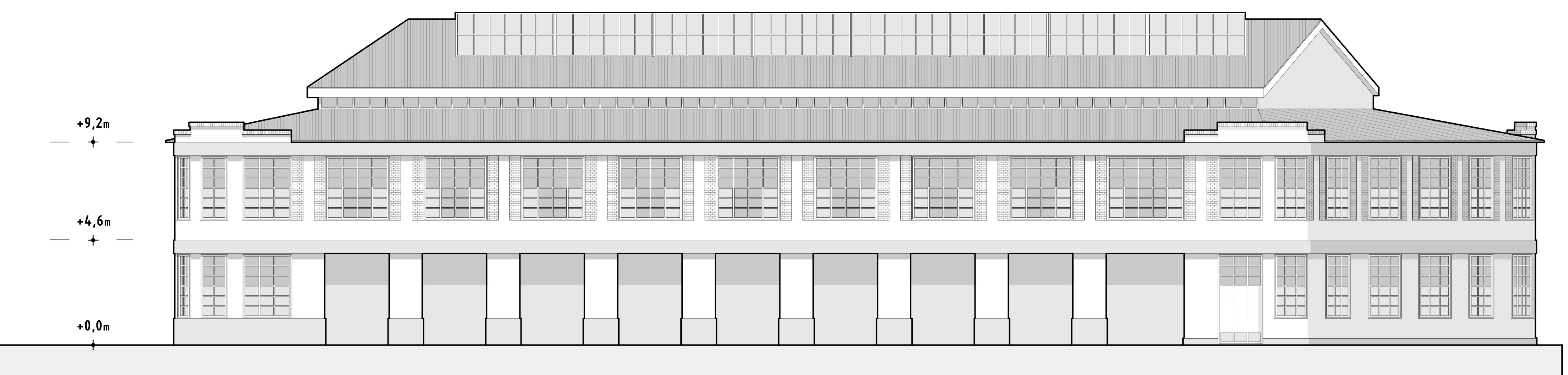
Portugaleteko Merkataria mendebaldeko altxaera Eskala 1 : 250
