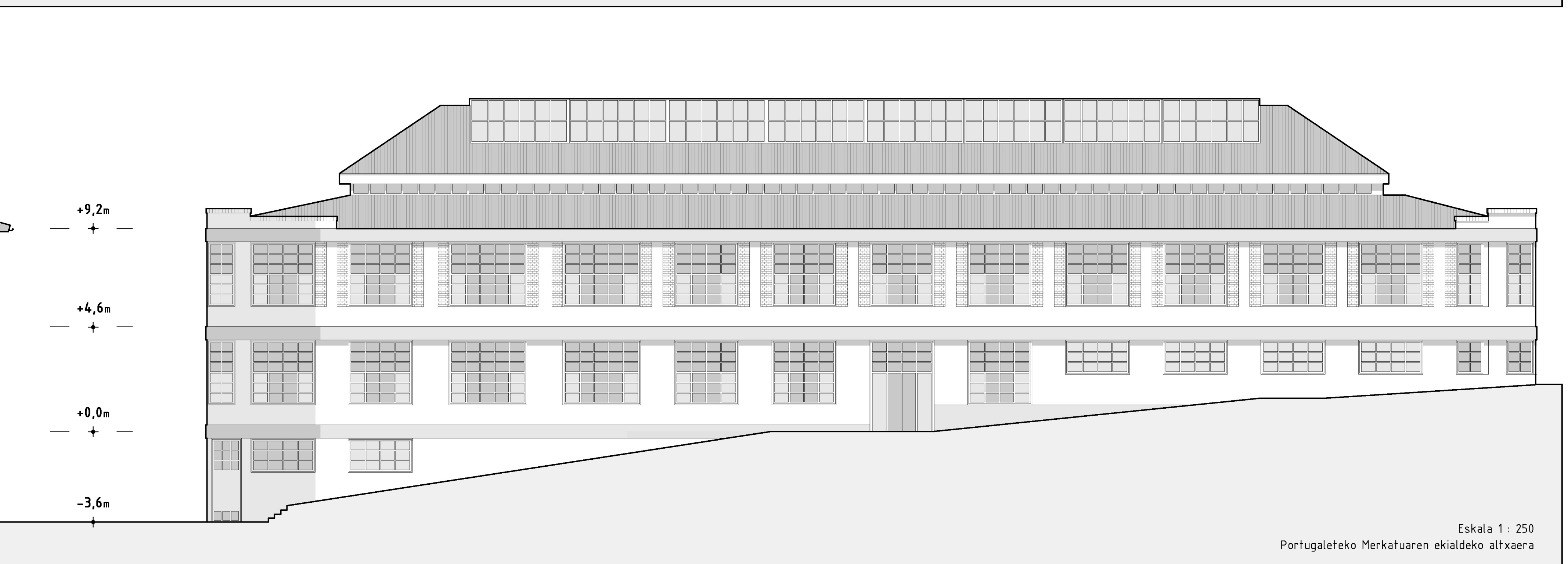
Portugaleteko Merkataria ekialdeko altxaera Eskala 1 : 250
