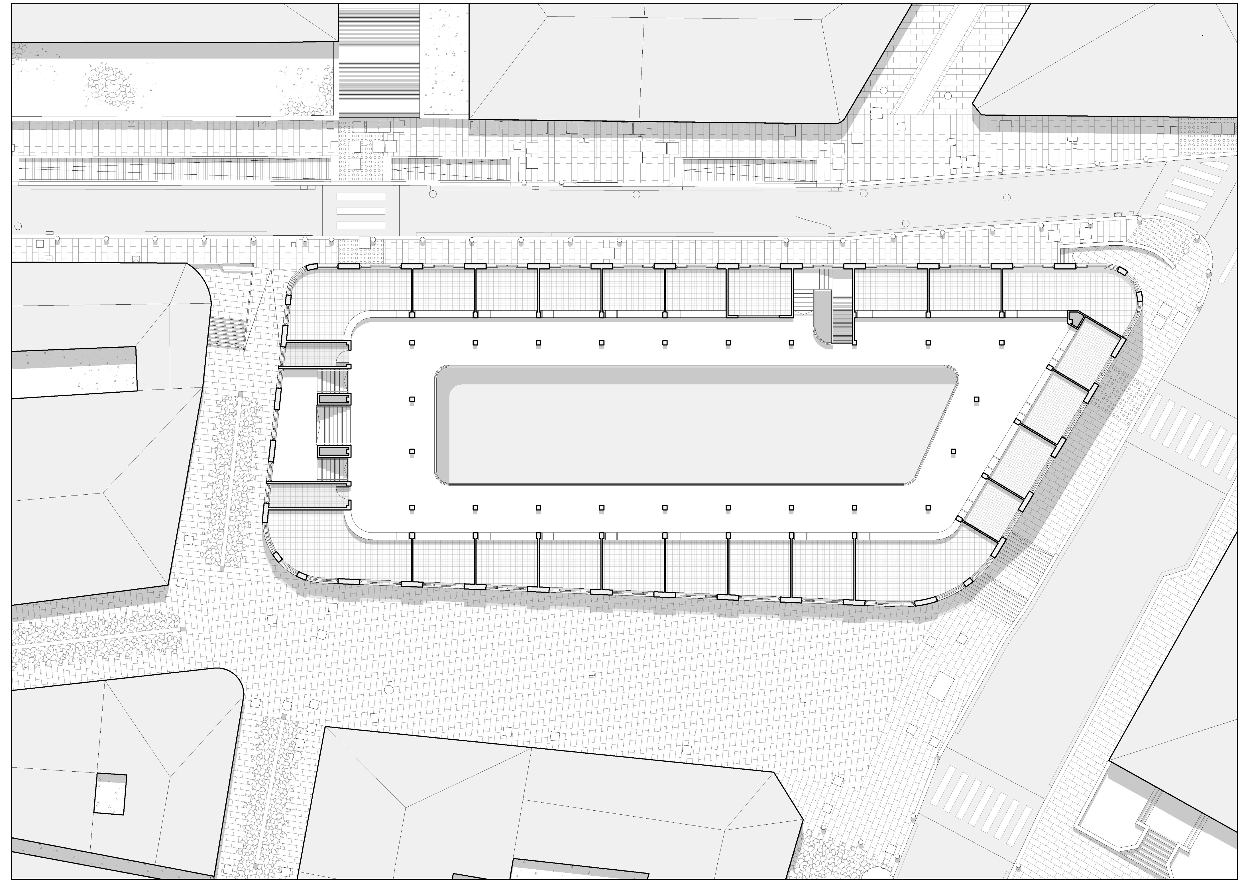
LEHENENGO SOLAIRUA Eskala 1 : 300 Portugaleteko Merkataria lehenengo solairua
