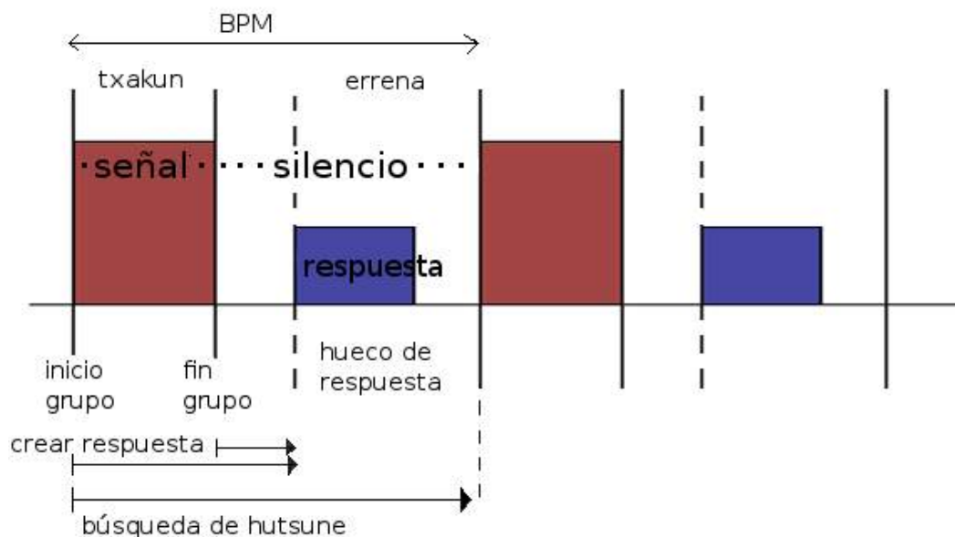
Gráfico 26: Estructura en el tiempo del algoritmo implementado.
