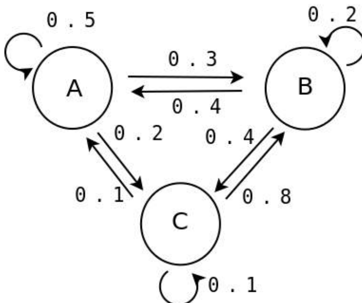
Gráfico 30: Gráfico descriptivo de las opciones de una cadena de Markov
