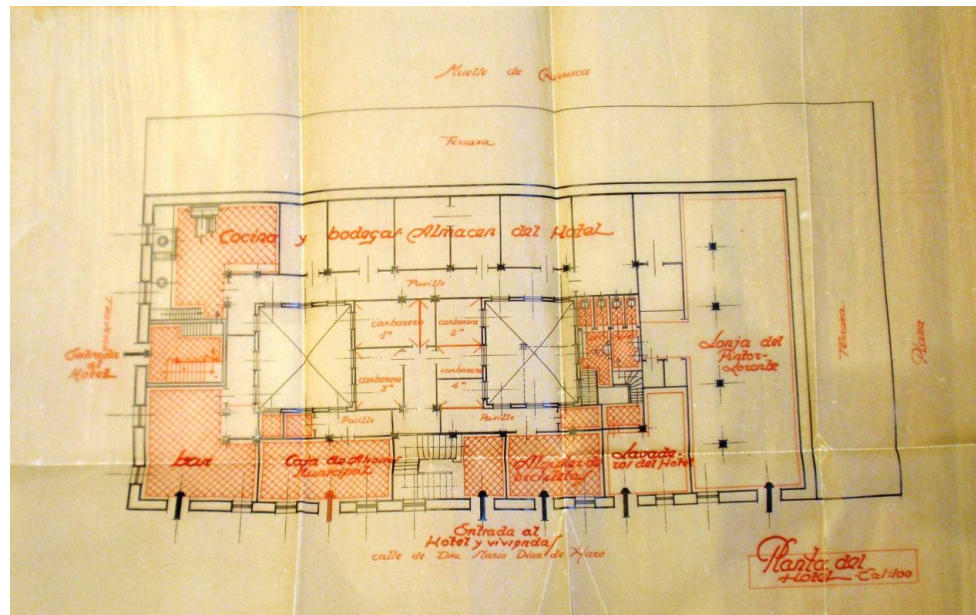
Imagen 13. Planta baja del hotel, según una propuesta de reforma de Santos Zunzunegui (1938).
