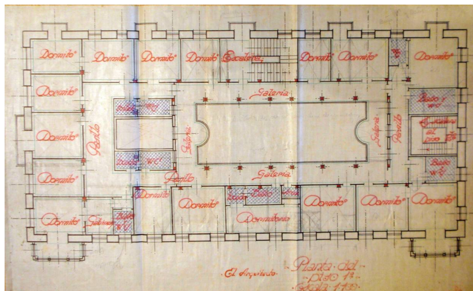
Imagen 16. Segunda planta del hotel, según la propuesta de reforma de Santos Zunzunegui (1938).
