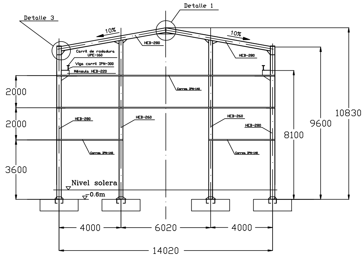
Pórtico hastial delantero
