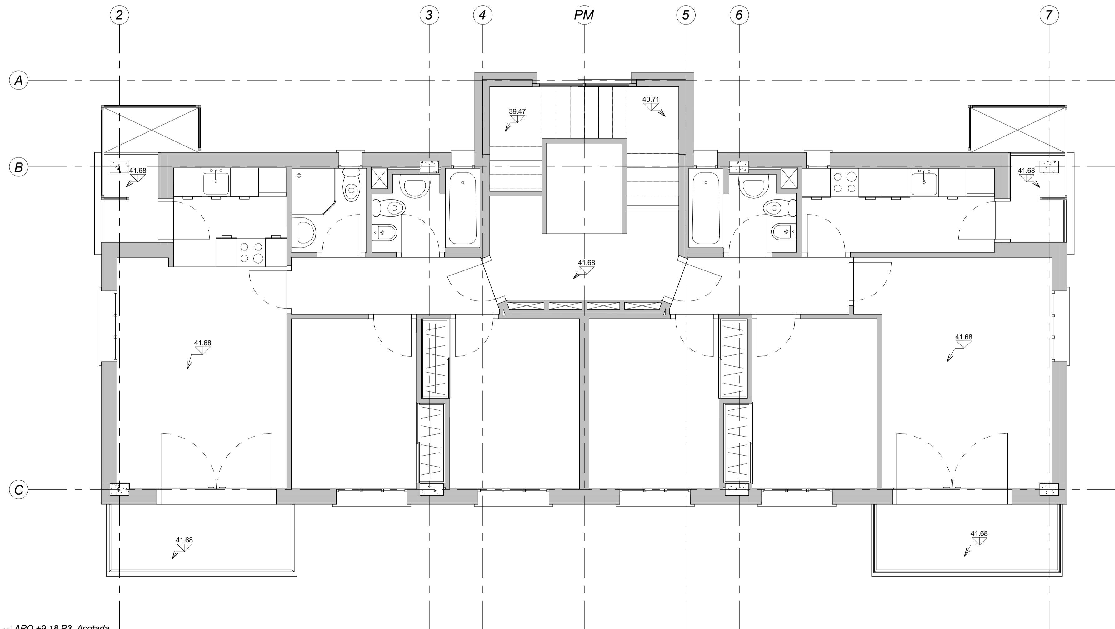
ARQ-05 | ARQ +9.18 P3 Acotada 1:50
