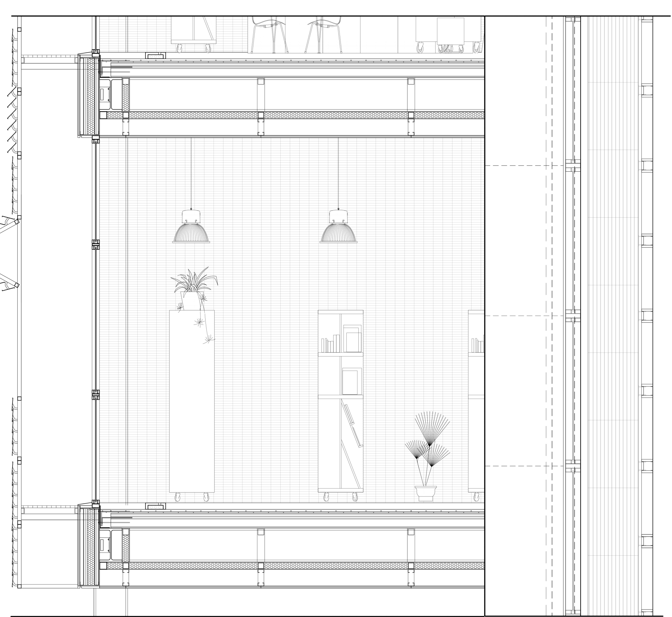
Beirako Fatxada detaila E1/30 Fatxada detaila linean E1/30
