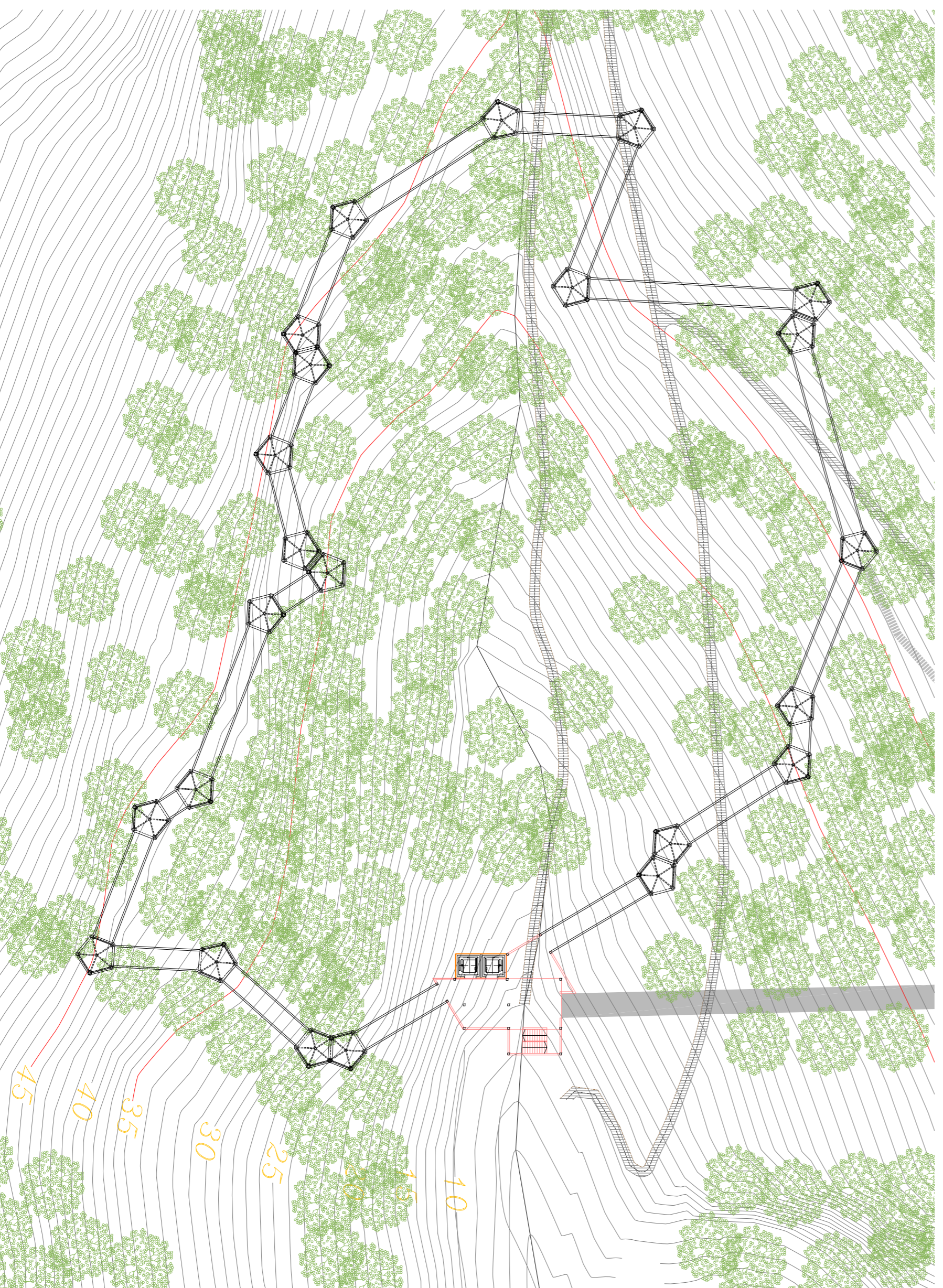
PLANTA DE CONJUNTO
