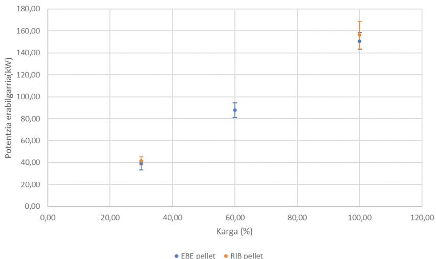
Galdarak emandako potentzia erabilgarria
