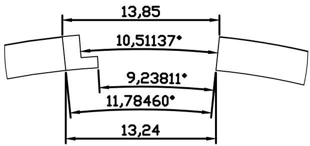
DETALLE D ESCALA 3 : 1
