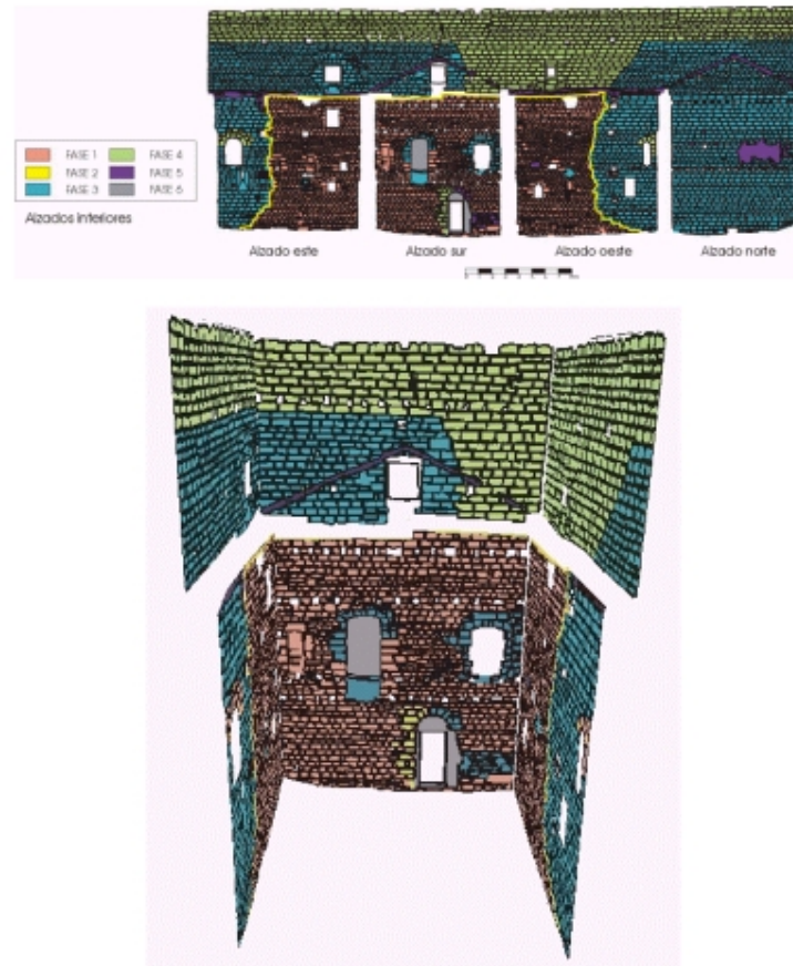
Figura 8.- Estudio histórico representado sobre los alzados y remontado como modelo virtual (interior de la Torre de Martiartu, Erandio, Bizkaia).
