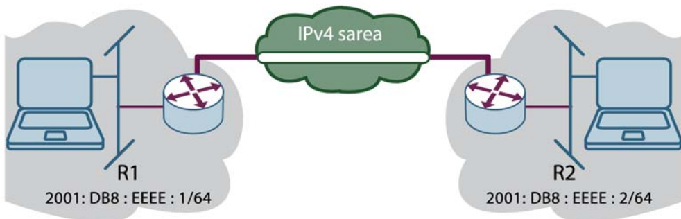
7. IRUDIA. IPv6 SAREAK ZEHARKATZEKO ESKUZO TUNEL BATEN FUNTZIONAMENDUAREN ESKEMA
