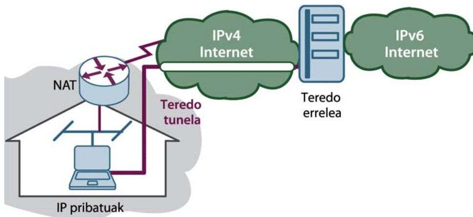
9. IRUDIA. TEREDO/MIREDO TUNELEN FUNTZIONAMENDUAREN ESKEMA
