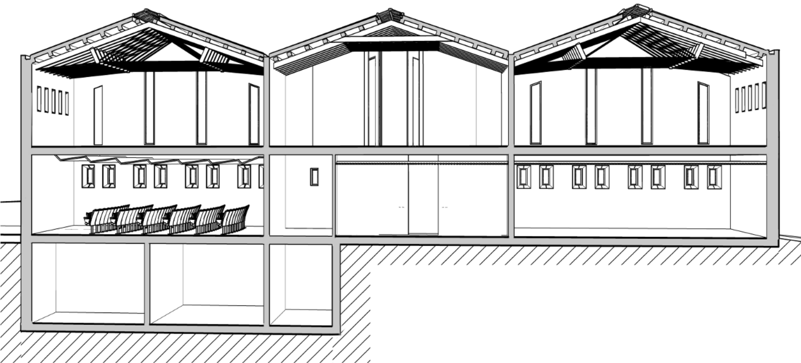
SECCION B-B
