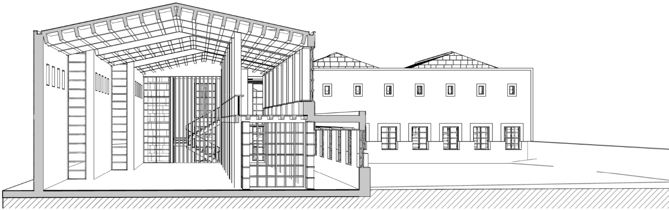
SECCION A-A
