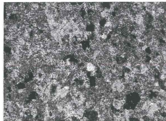
FOTO 8. Aspecto microscópico de sílex pertenecientes a formaciones asociadas a basaltos del sinclínorio vizcaíno donde se observa una textura relicto calcarenítica. Anchura del campo: 3 mm. Luz polarizada.
