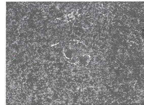
FOTO 9. Aspecto microscópico de sílex costero de grano fino donde se observa un foraminífero ( Rotalido ) y una importante alteración que opacifica la textura silíceo. Anchura del campo: 3 mm. Luz polarizada.
