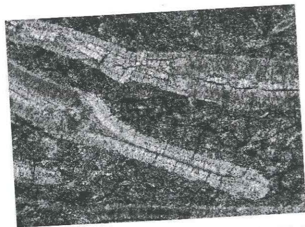
FOTO 6. Detalle microscópico de Nummulitidos del género Operculina perteneciente a sílex del Terciario marino de Urbasa. Anchura del campo: 3 mm. Luz polarizada.
