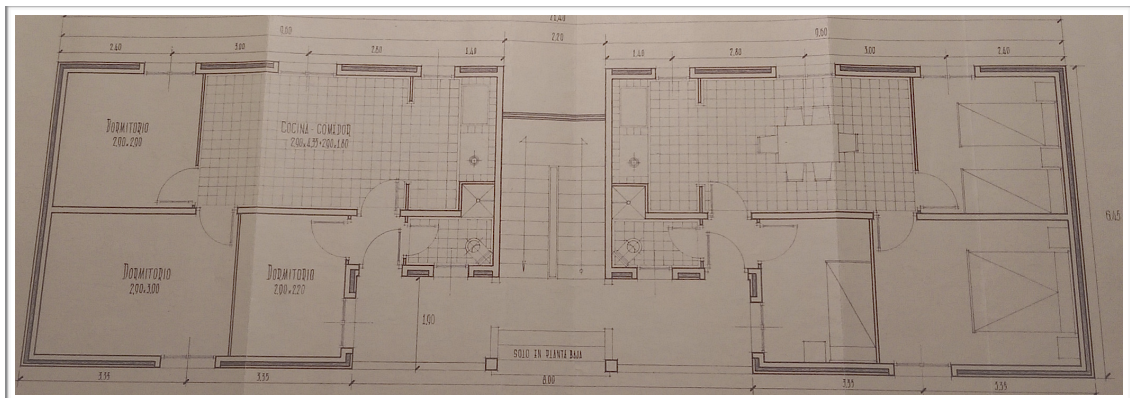
Ilustración 11:Plano de planta de las viviendas 1958 (Fuente: AMVG 45/33/9)
