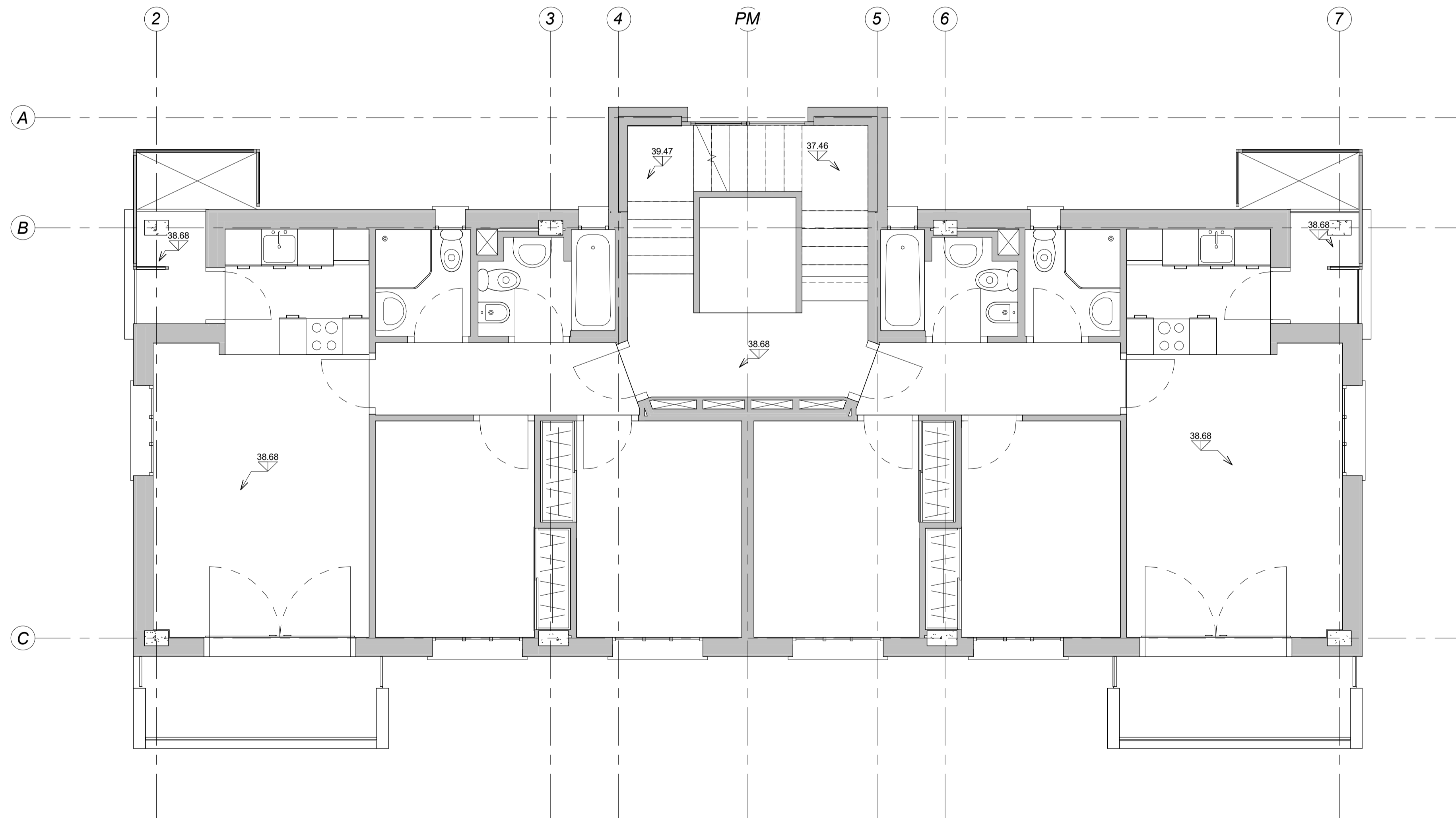
ARQ-04 ARQ +6.18 P2 Acotada 1:50
