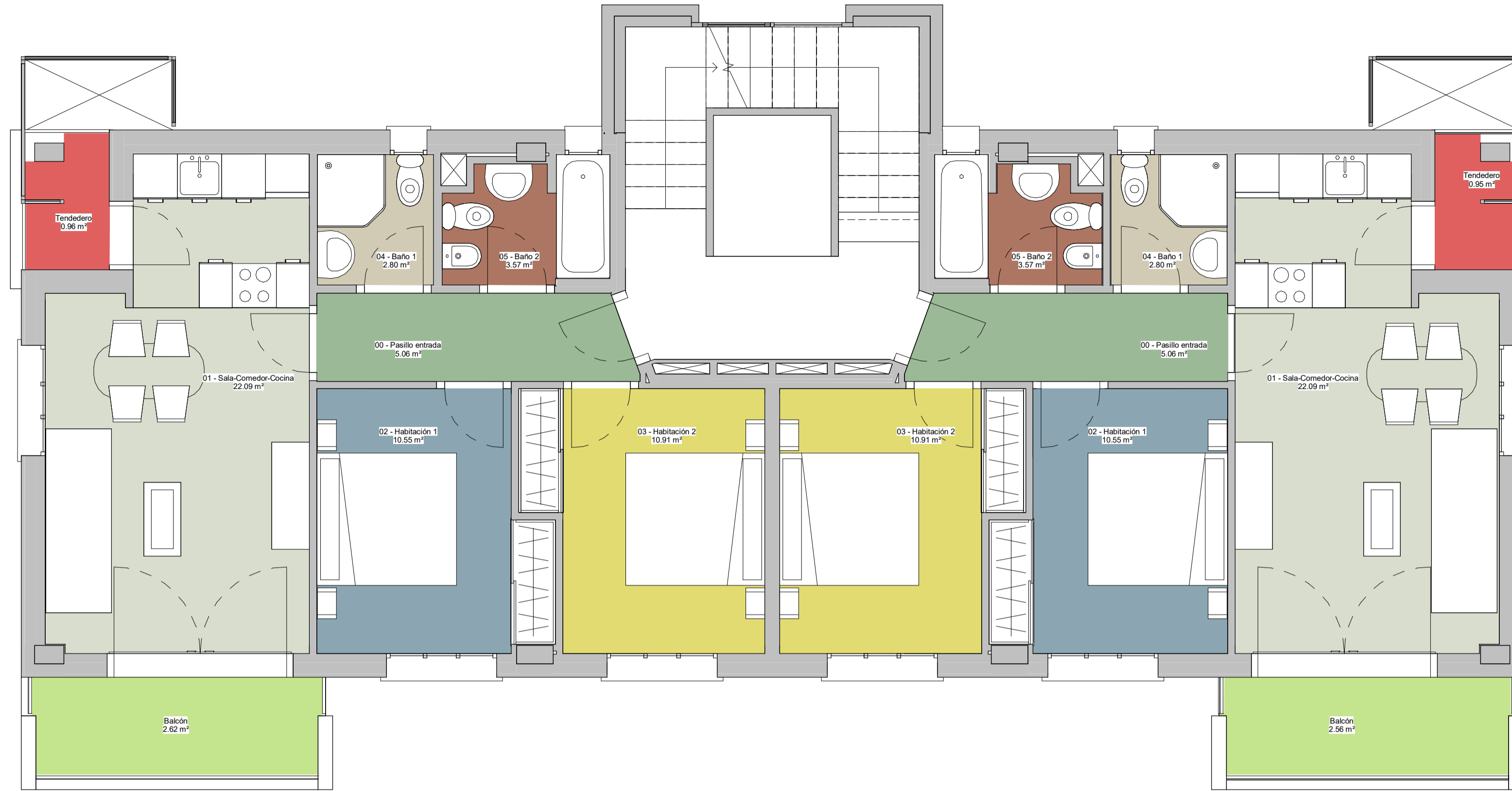
ARQ-09 ARQ+6.18 P2 1:50
