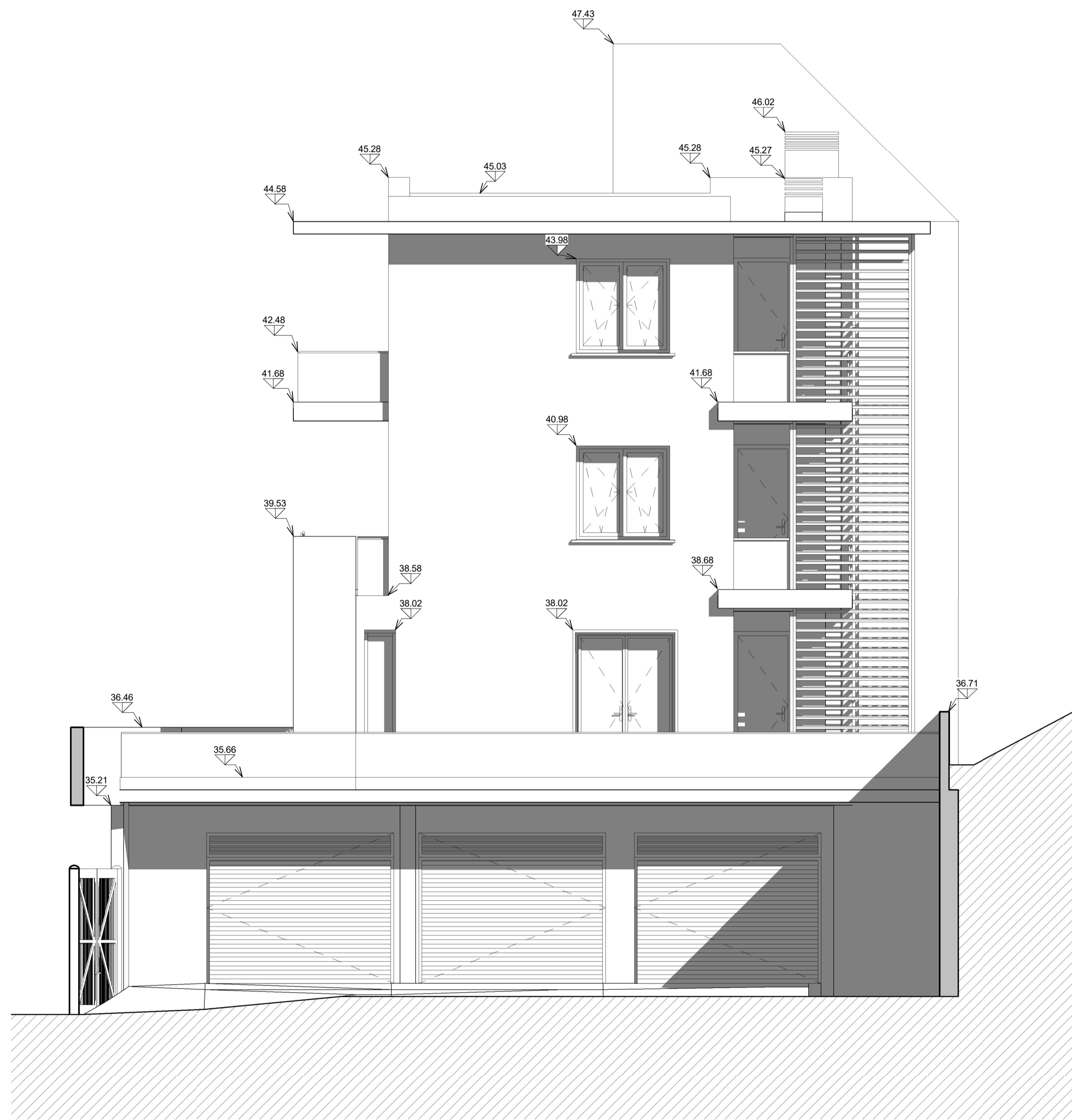
ARQ-14 Este 1:50
