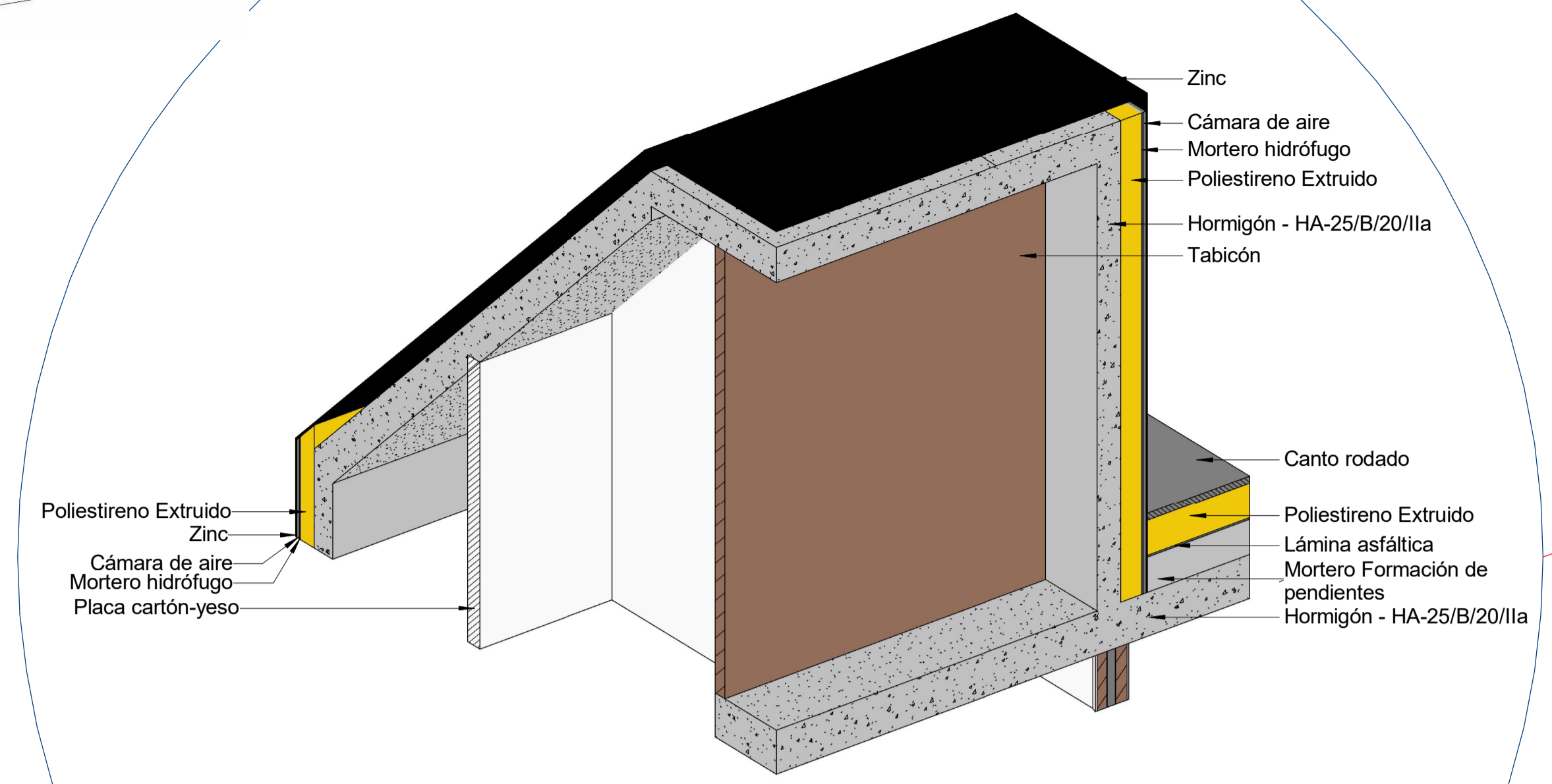
ARQ-20 Encuentro cubierta con caja de ascensor
