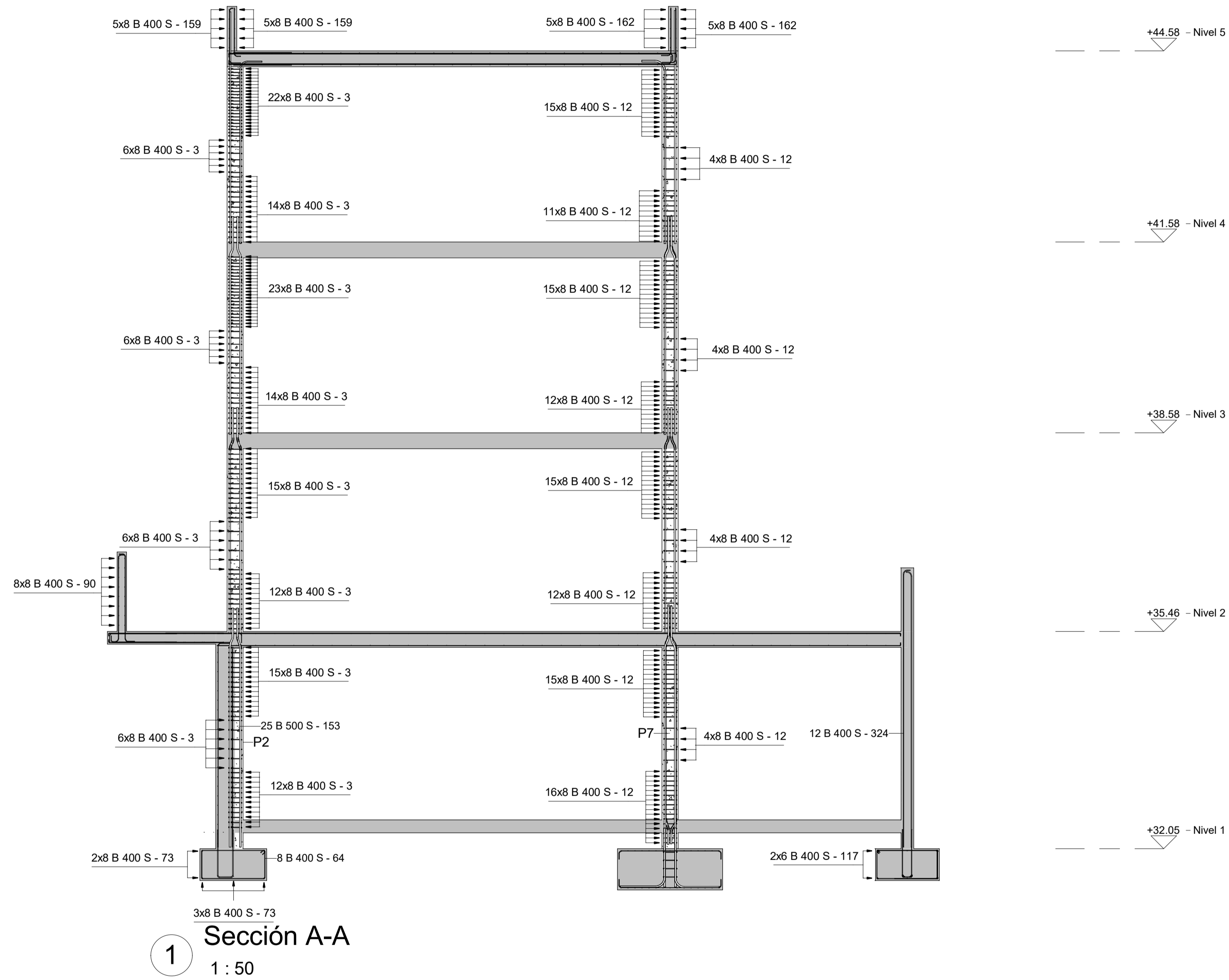
CML_PILARES ESTRUCTURALES_PB
