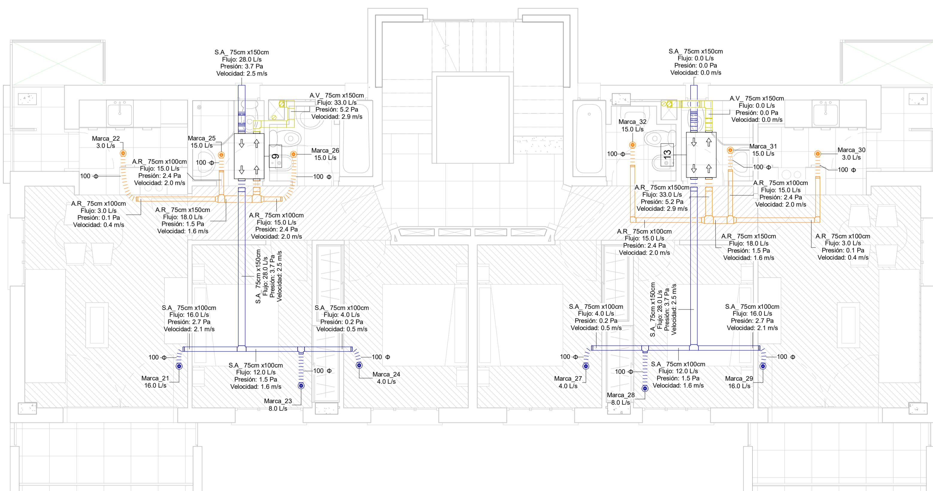
1 Ventilación P2 1 : 50
