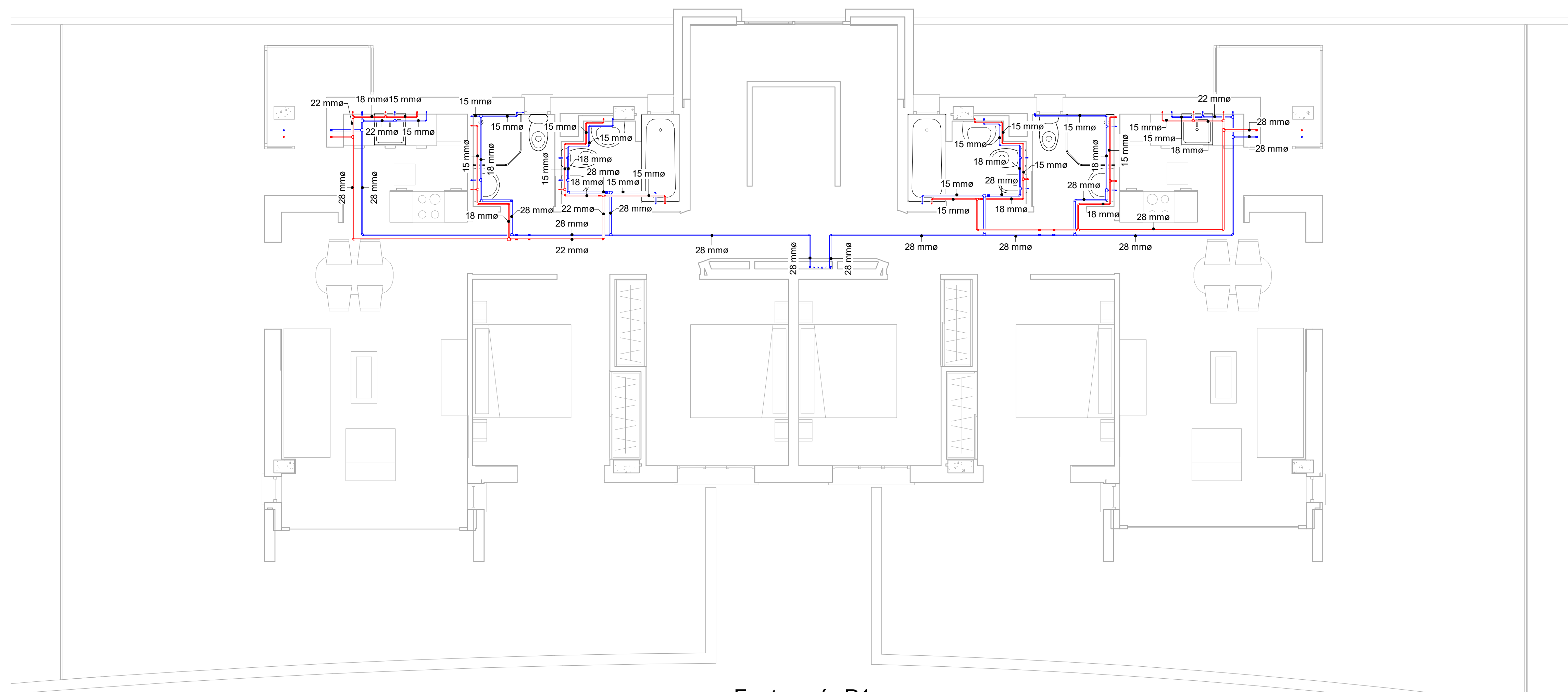
1 Fontanería P1 1 : 50
