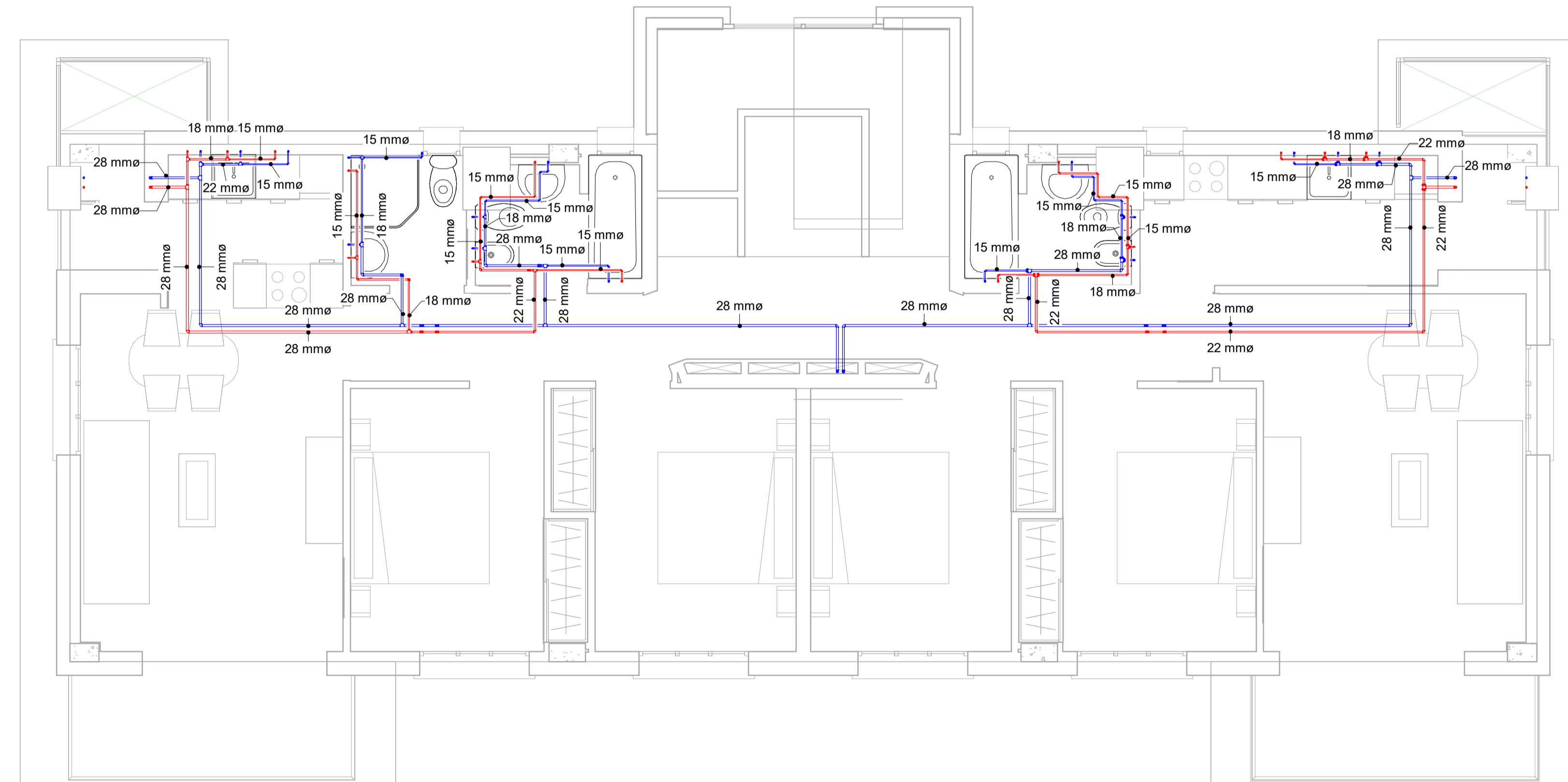
1 Fontanería P3 1 : 50
