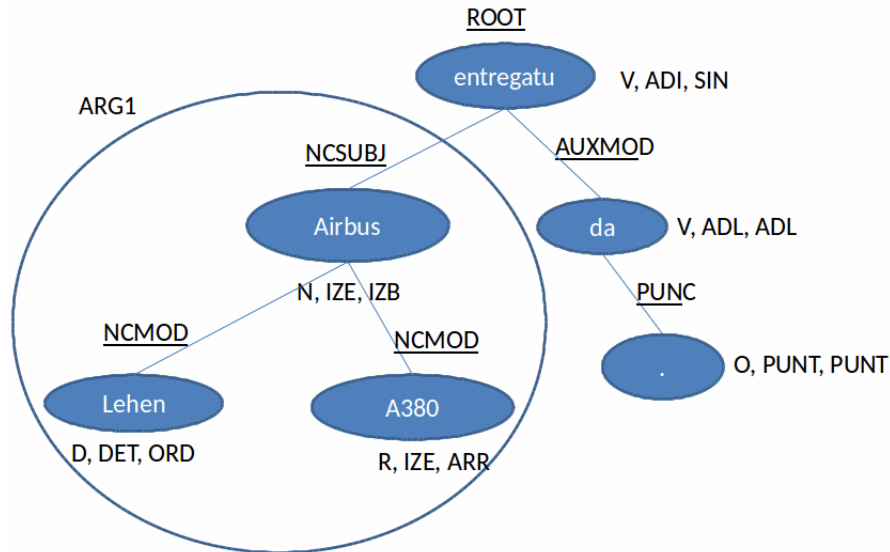
5.8 irudia – Lehen Airbus A380 entregatu da esaldiaren dependentzia-zuhaitza
