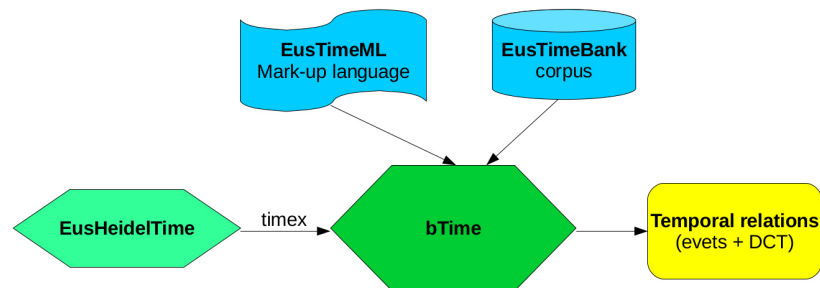
5.24 irudia – bTime sistemaren arkitektura
